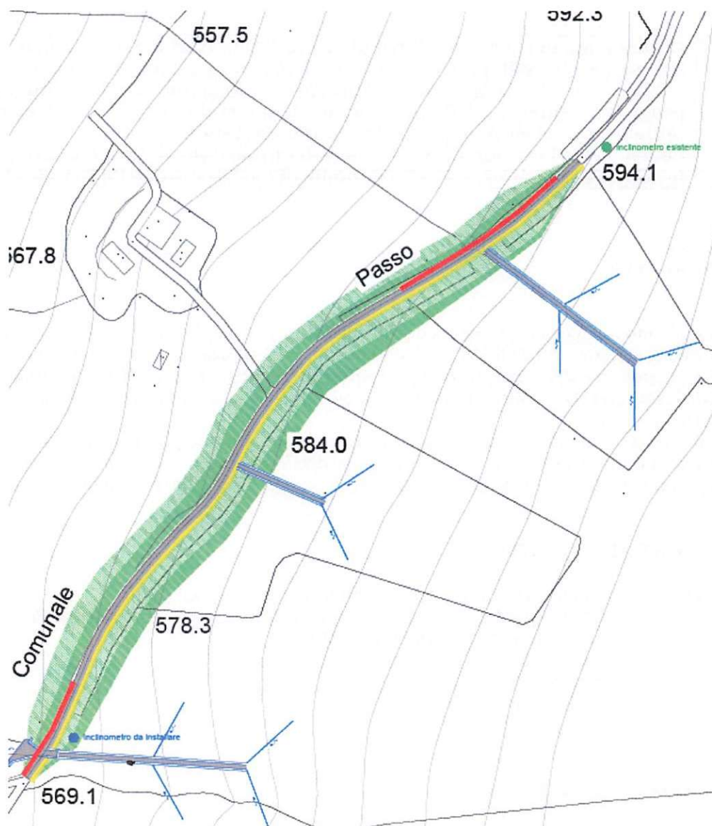
Figura 1 - Mappa recante l'ubicazione dell'installazione inclinometrica
